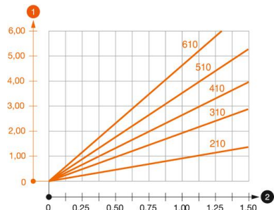
Диаграмма нагрузки на кронштейн типа AW 15
