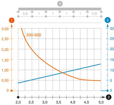
Диаграмма нагрузки на кабельный лоток лестничного типа, тип LG 110 VS
