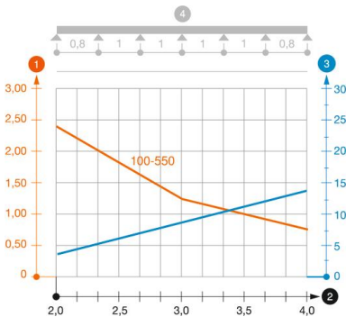
Диаграмма нагрузки на кабельный лоток типа SKSMU 110
