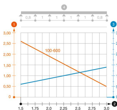
Диаграмма нагрузки на кабельный лоток типа SKSMU 60
