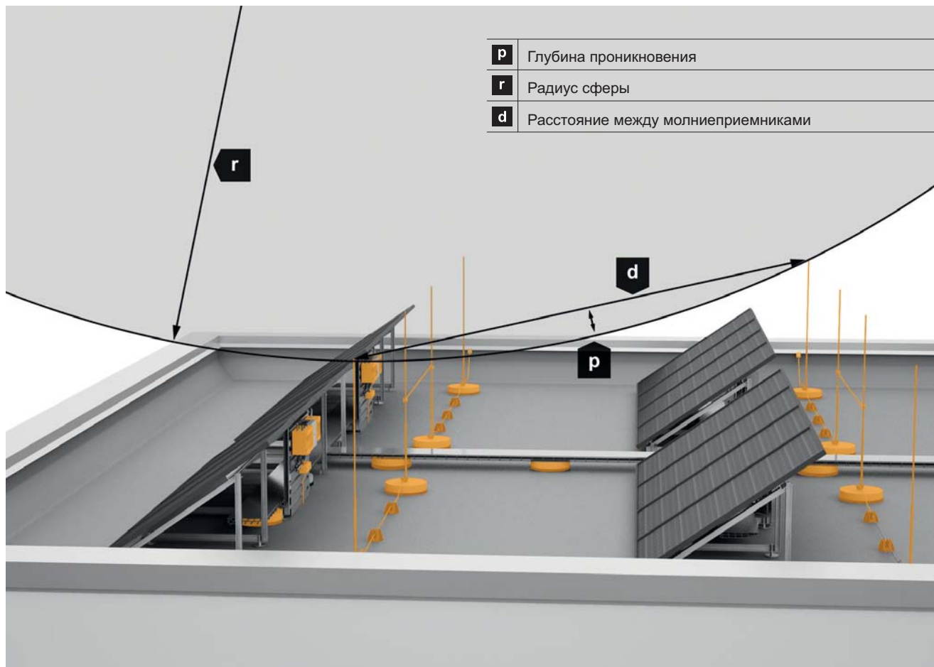
Рис. 2.8: Глубина проникновения (p) сферы между молниеприемными стержнями
