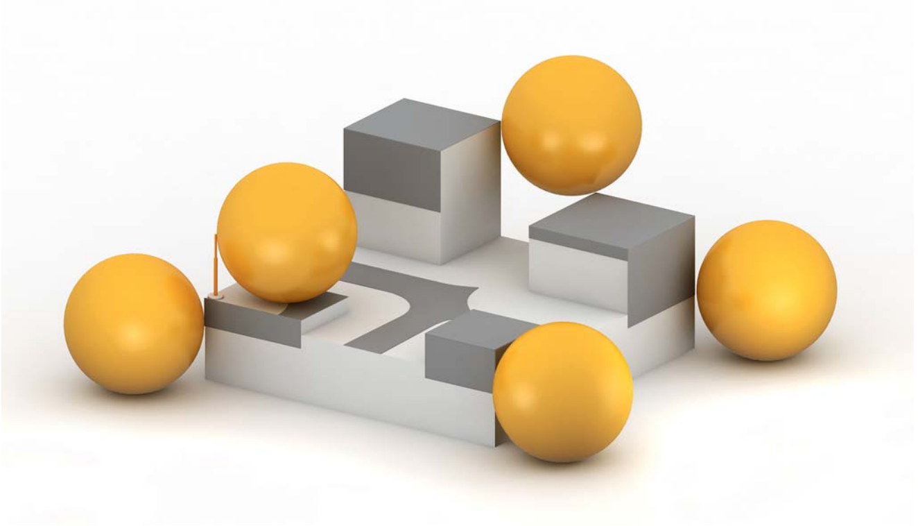
Рис. 2.4: Рис. 2.6: Метод скатящейся сферы (темно-серые участки находятся под угрозой удара)
