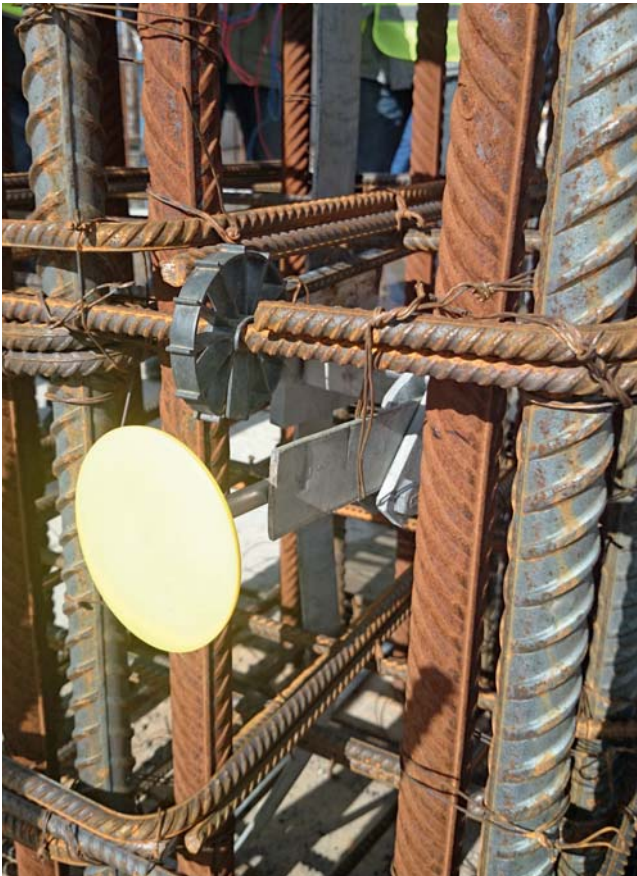
Пример крепления опорной точки заземления к плоскому проводнику перед заливкой фундамента общественного делового комплекса «Лахта-Центр», г. Санкт-Петербург, Россия
