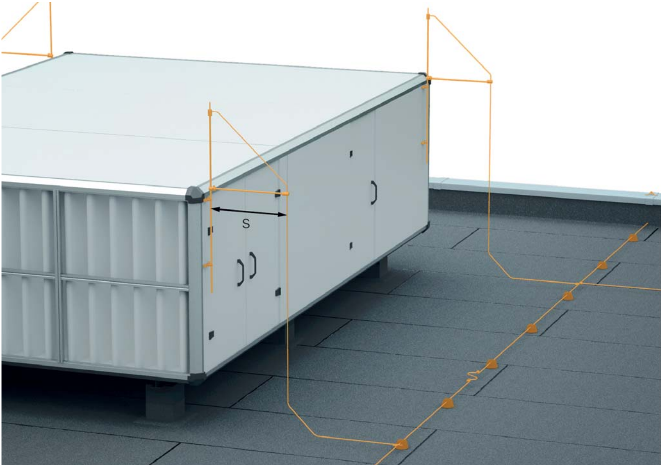
Рис. 2.17: Соблюденный разделительный интервал ( s ) между токоотводными устройствами и кровельными
