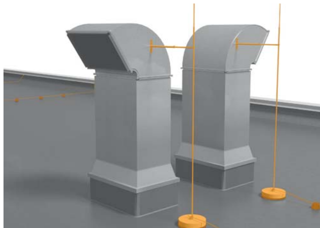
Рис. 2.31: Молниеприемный стержень с регулируемым дистанционным держателем
