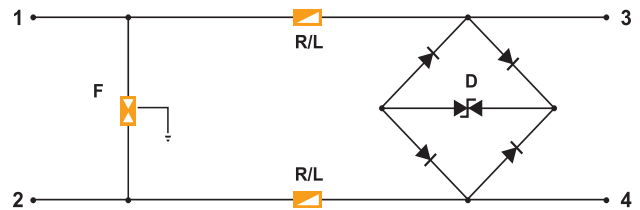
Рис. 3.67: Схема базовой защиты в измерительной цепи
