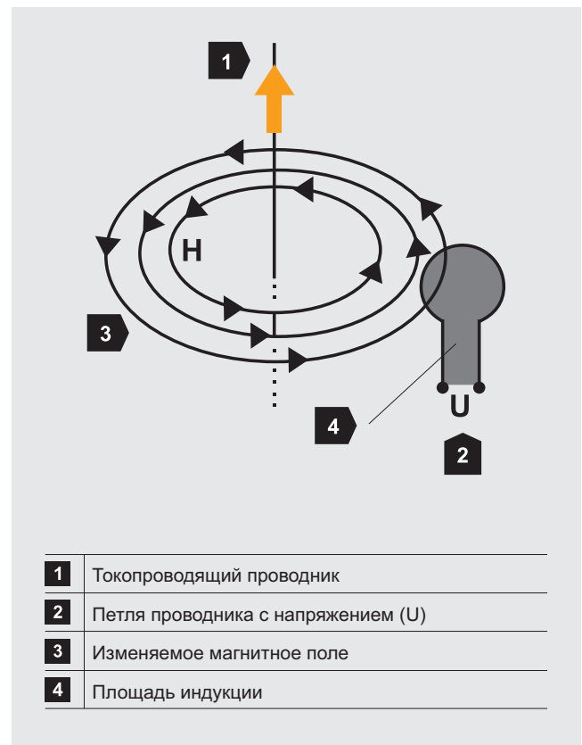
Рис. 3.41: Индукция в петле проводника
