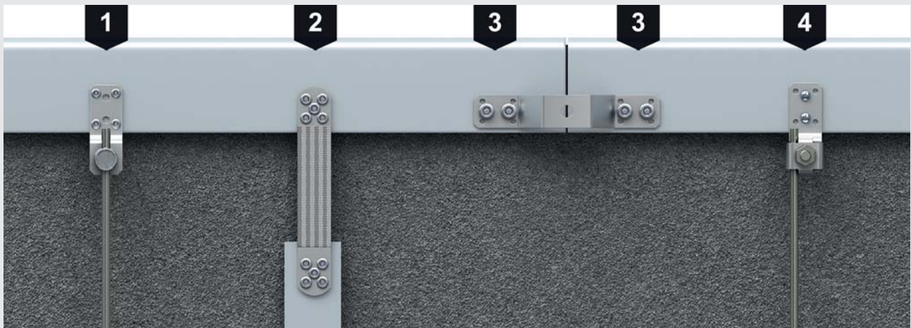
2.16: Примеры соединения металлического защитного ограждения
