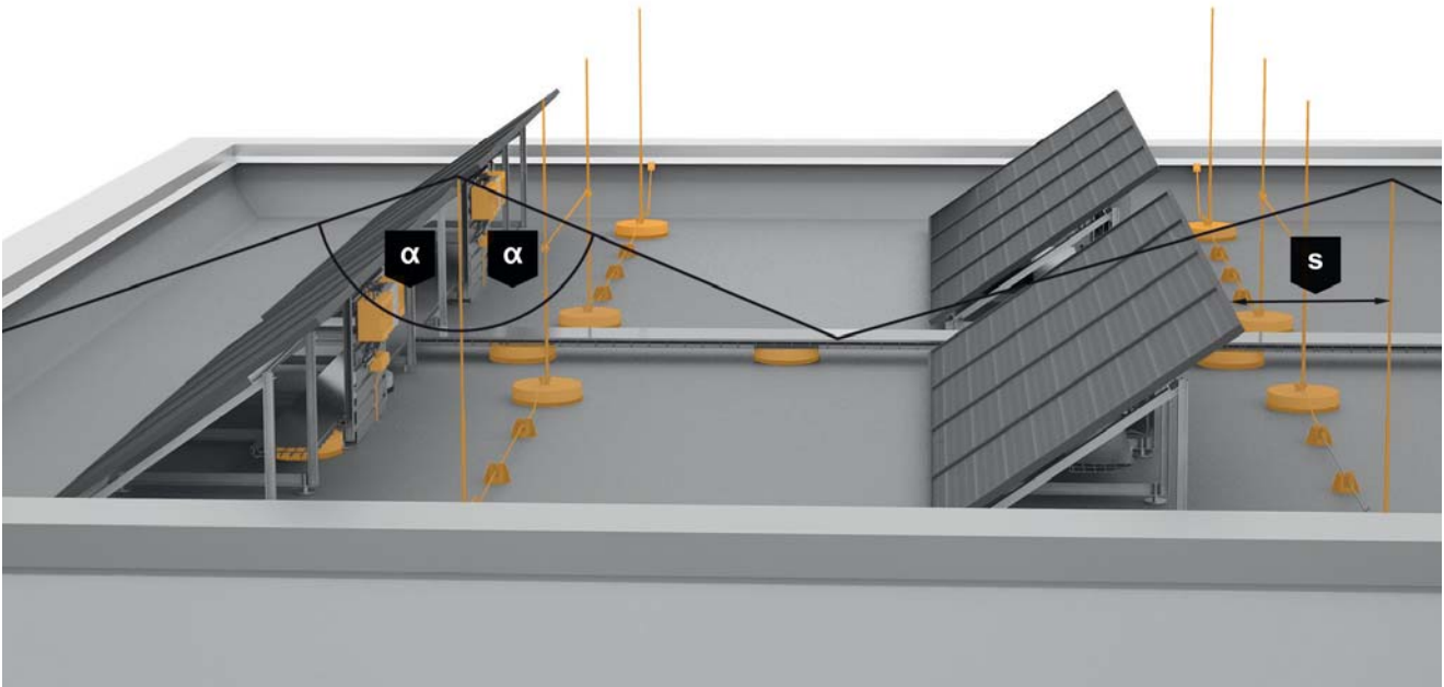
Рис. 2.9: Защитный угол и разделительный интервал на фотогальванической установке
