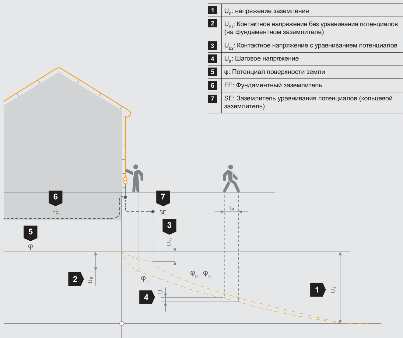
Рис. 2.94: Потенциал поверхности земли и напряжения при обтекаемом током фундаментном заземлителе ФЗ и заземлителе уравнивания потенциалов
