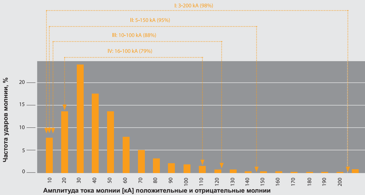
Рис. 1.20: Параметры тока молнии в соответствии с уровнем угрозы (уровнем молниезащиты) LPL согласно ГОСТ Р МЭК 62305-1-2010
