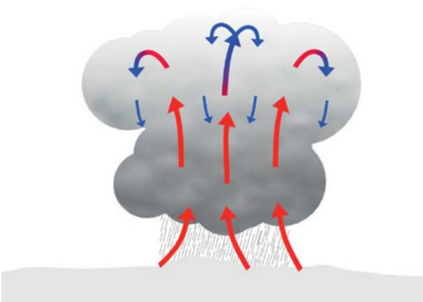
Рис. 1.4: Тепловая гроза
