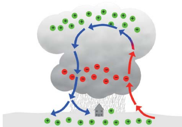
Рис. 1.5: Возникновение молнии – отрицательные и положительные заряды
