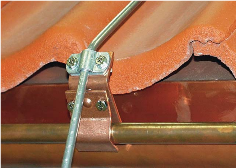
Рис. 2.96: Биметаллический держатель проводника для водосточных желобов (алюминиевый круглый проводник и медный водосточный желоб)
