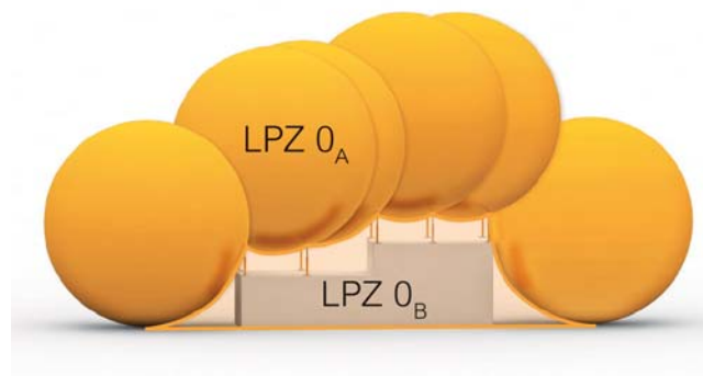
Рис. 2.5: Метод катящейся сферы и вытекающие из него зоны молниезащиты (LPZ)
