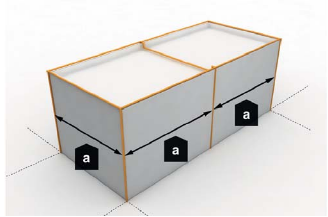
Рис. 2.47: Расстояние (a) между токоотводами
