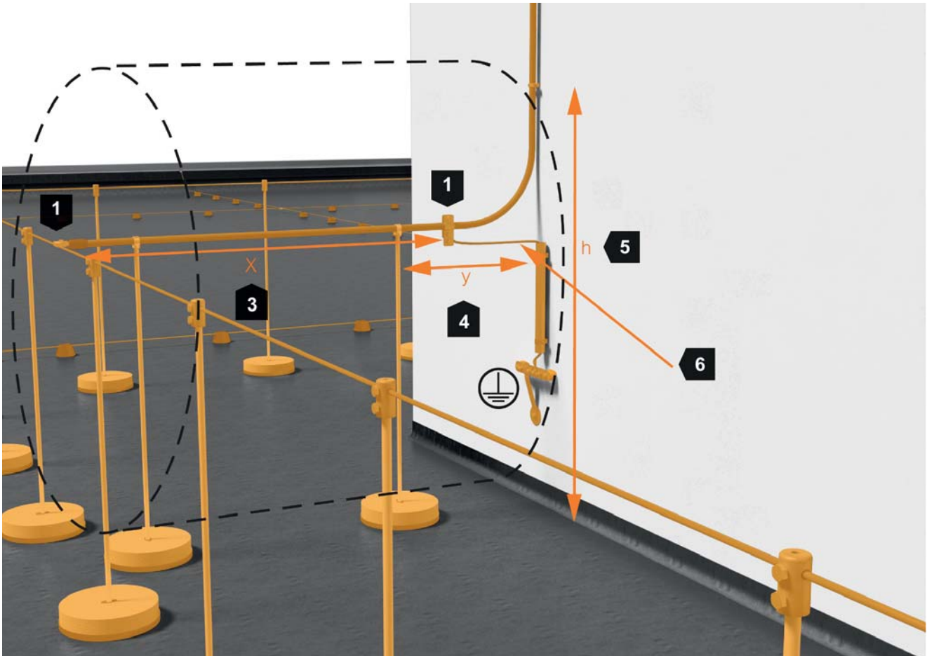
Рис. 2.69: Пример монтажа системы с токоотводом isCon
