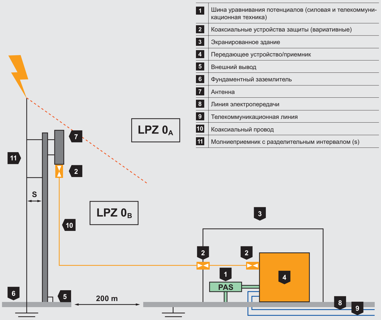
Рис. 3.78: Изолированная молниезащита на антенной установке и в различных системах заземления 200 м
