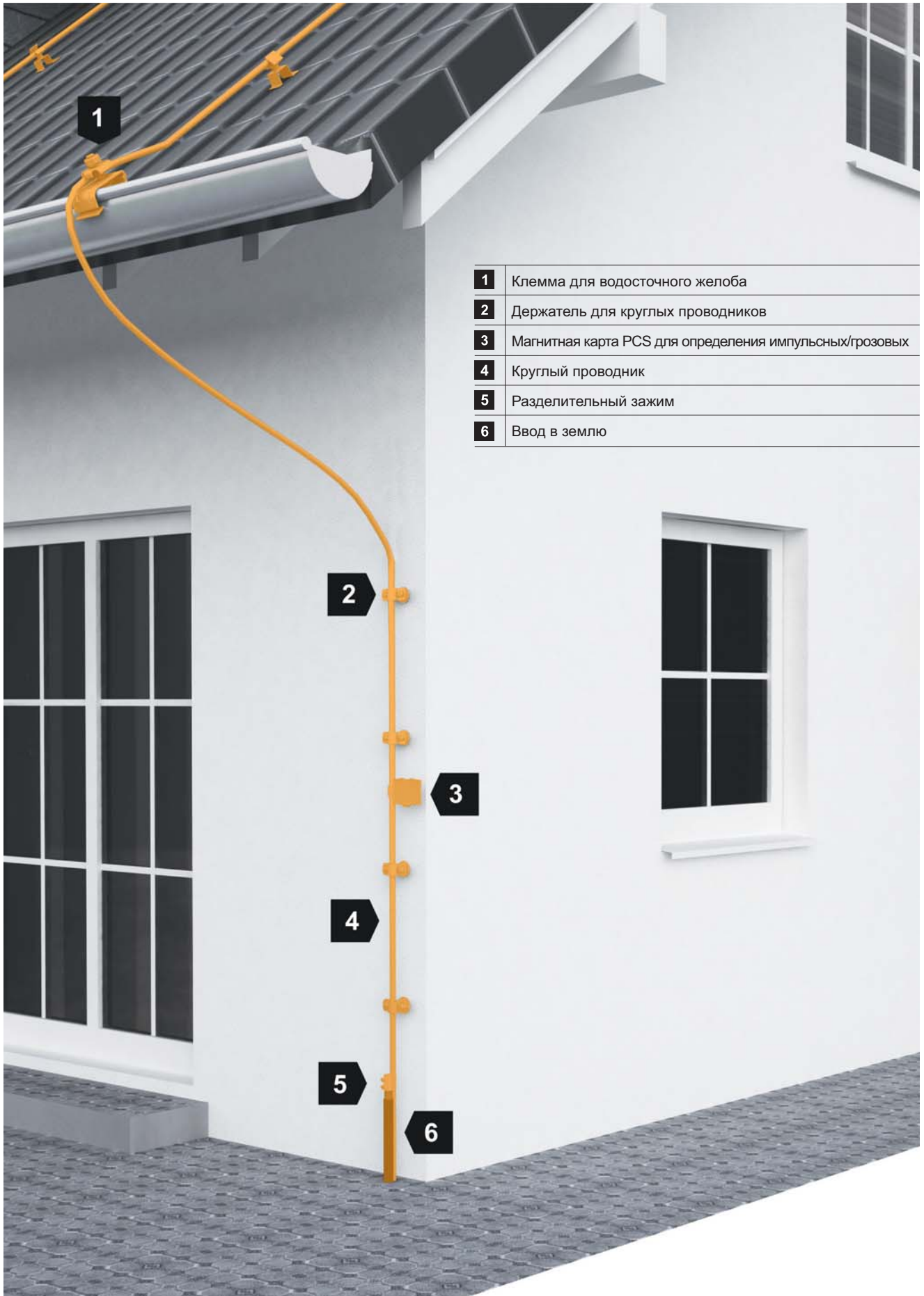
Рис. 2.50: Принцип монтажа токоотвода
