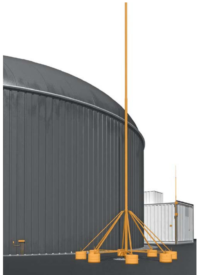
Рис. 2.30: Телескопические молниеприемные мачты irod: применение для установки, работающей на биогазе
