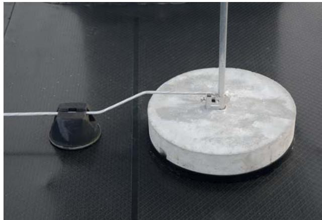
Рис. 2.21: Молниеприемный стержень с опорной ножкой
