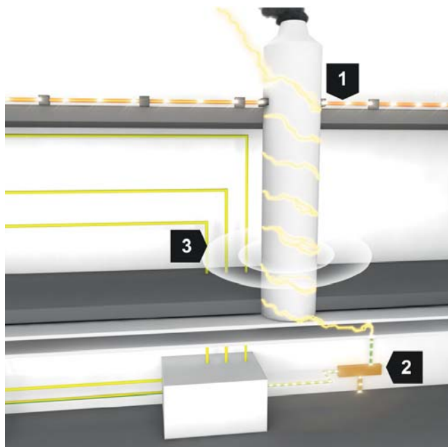
Рис. 2.22: Изолированная молниезащита с молниеприемной мачтой isFang
