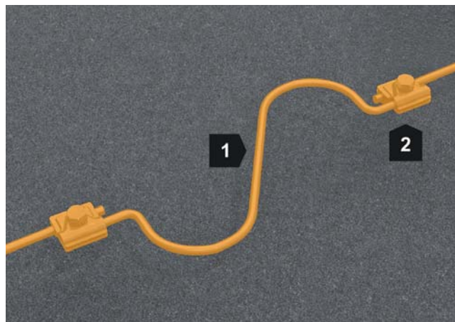
1 Компенсатор температурного расширения 2 Зажим
