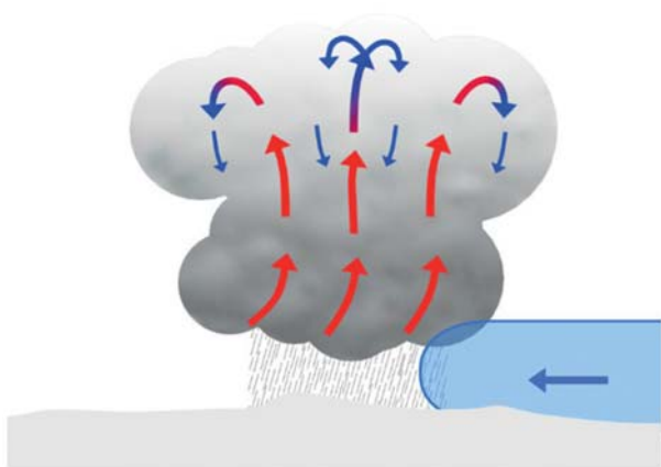
Рис. 1.3: Холодный воздушный фронт
