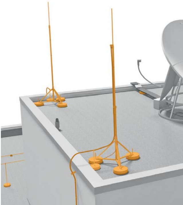
Рис. 2.26: Молниеприемные мачты с расположенным снаружи токоотводом isCon®
