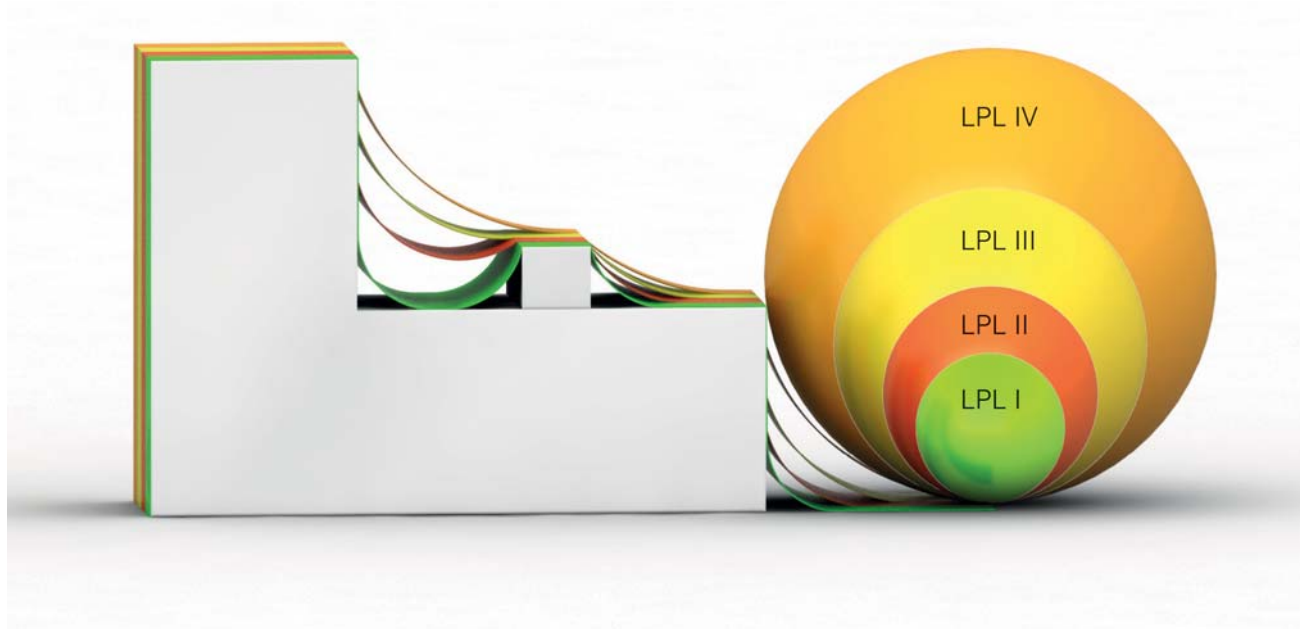
Рис. 2.4: Радиус сферы молнии в зависимости от класса молниезащиты
