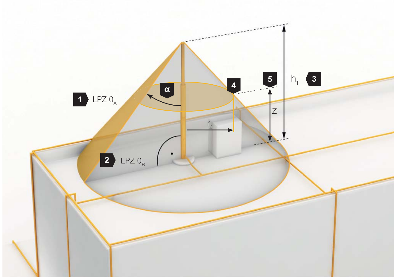
Рис. 2.10: Рассчитанная на основе упрощенного метода защитного угла защитная площадь молниеприемного стержня.
