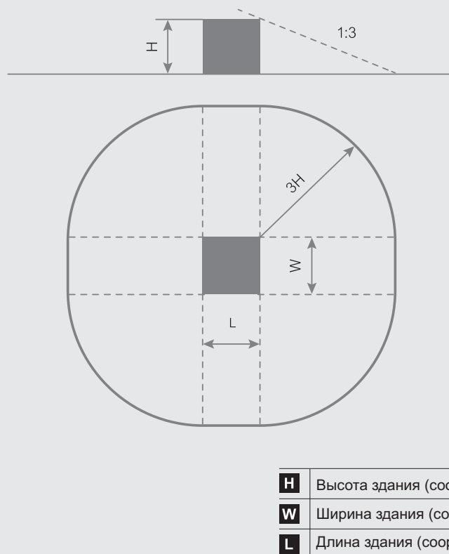
Рис. 1.22: Пример определения области защиты от прямых ударов молнии
