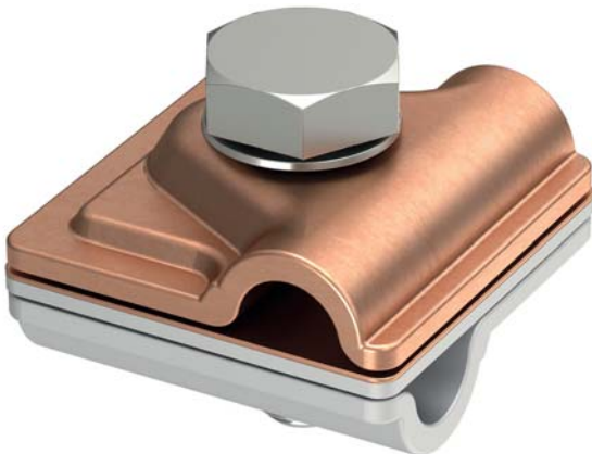
Рис. 2.95: Биметаллический быстроразъемный соединитель Varjo с биметаллической промежуточной пластиной (медь/алюминий)
