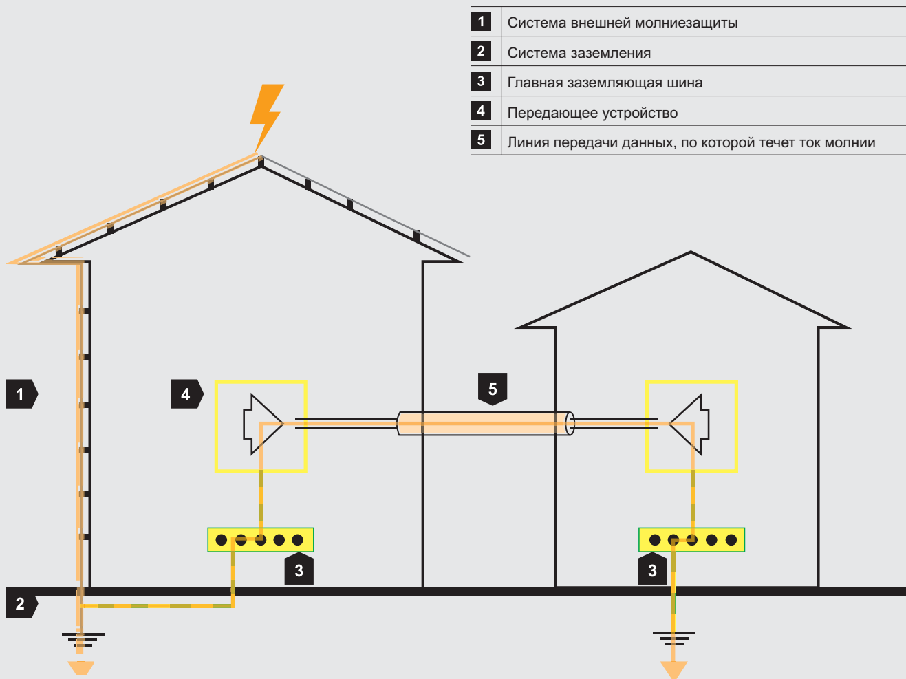
Рис. 3.36 Гальванический ввод в линию передачи данных через систему внешней молниезащиты
