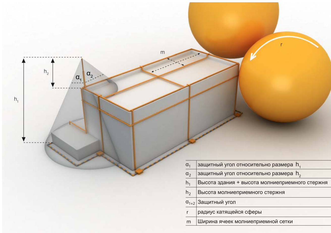
Рис. 2.2: Проектирование с использованием методов защитного угла, молниеприемной сетки и метода катящейся сферы
