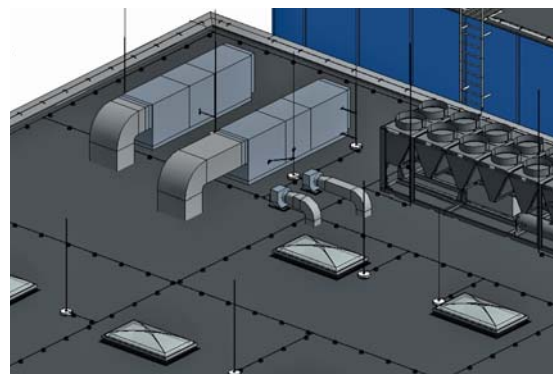
Рис. 6.2: Результат автоматической расстановки соединителей и держателей проводников
