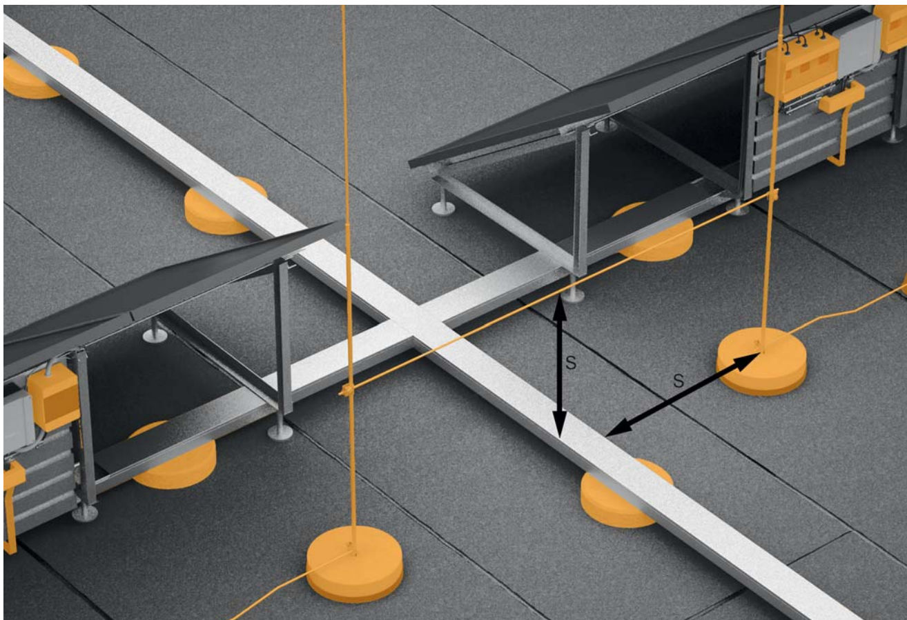
Рис. 2.20: Изолированная молниезащита с выполненным по нормам разделительным интервалом ( s )
