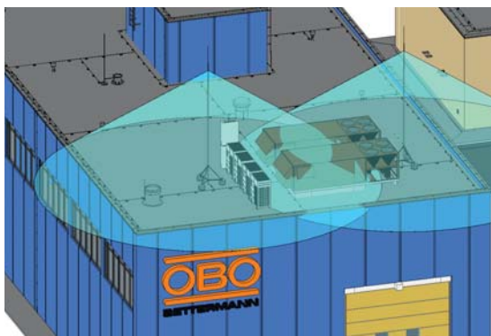
Рис. 6.1: Пример визуального отображения зоны защиты молниеприемников
