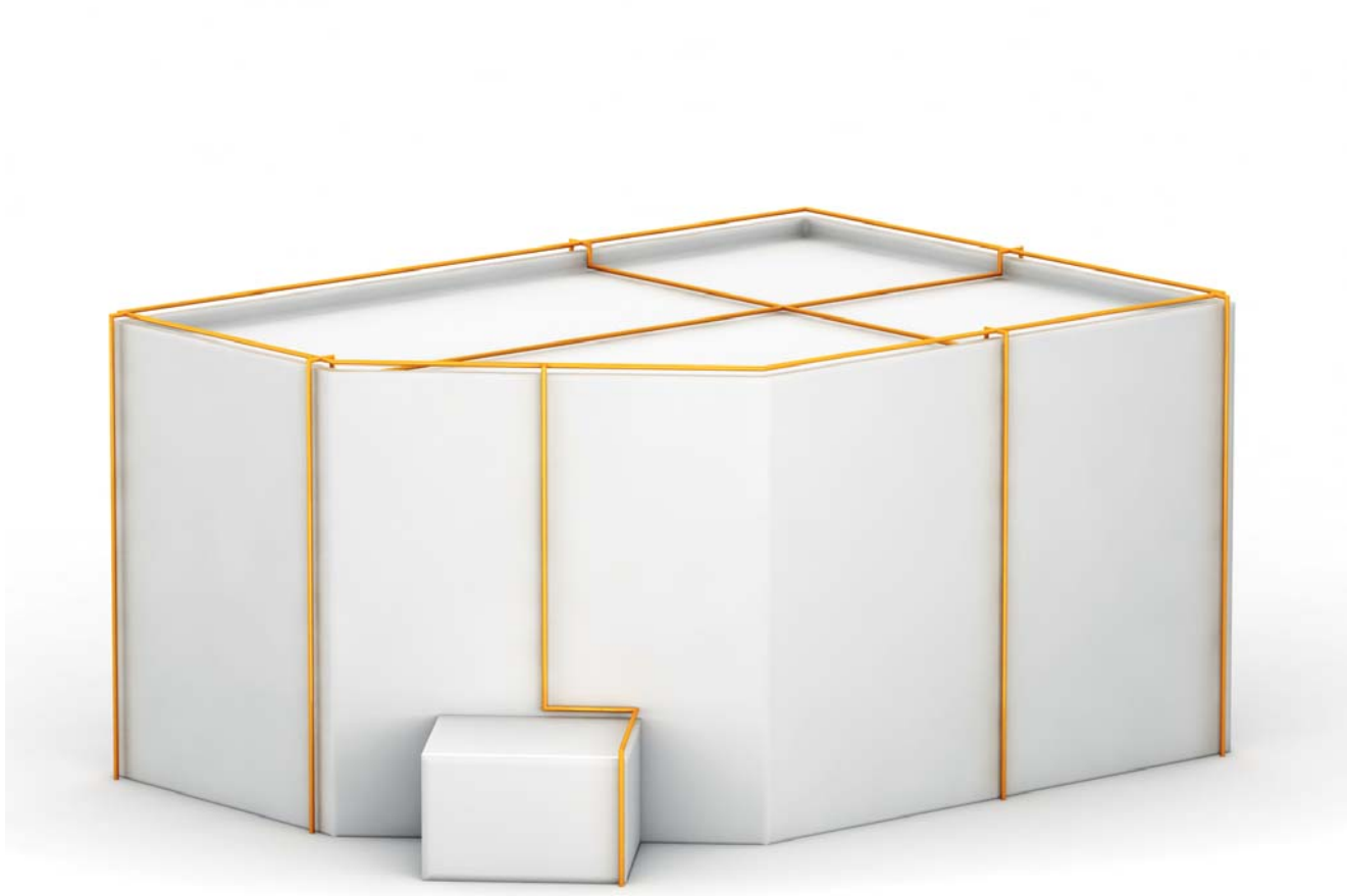
Рис. 2.46: Токоотвод в соответствии с МЭК 62305-3
