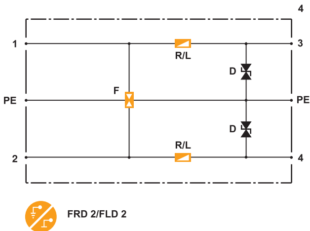
Рис. 3.66: Схема молниезащитного барьера FRD2/FLD2
