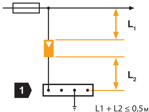
Рис 3.14: Максимальная длина ввода/вывода в соответствии с ГОСТ Р 50571.5.53
