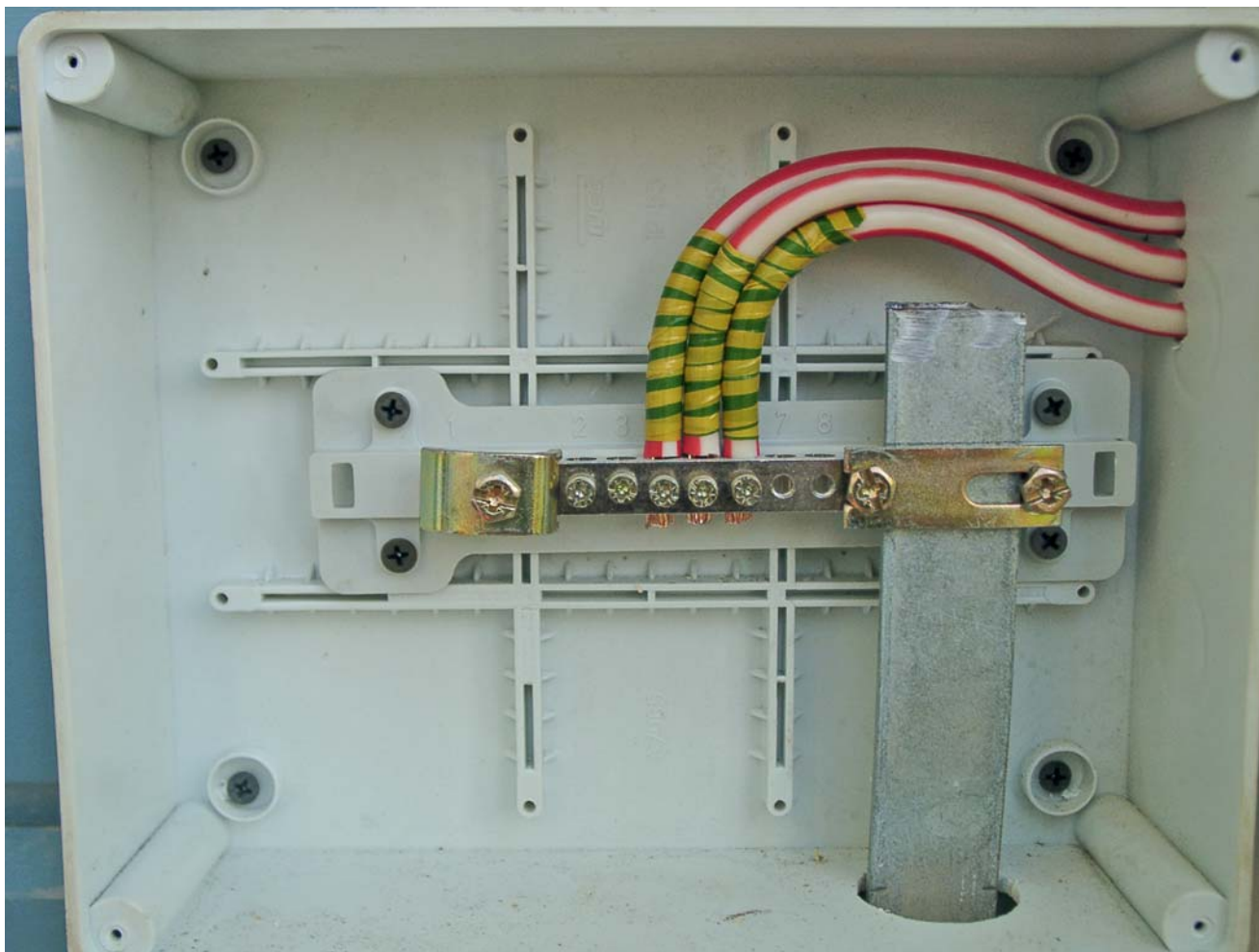
Полоса заземления и проводники системы уравнивания потенциалов подключаются к шине уравнивания потенциалов ОБО Беттерманн (верхняя крышка снята), Ленинградская область, Россия
