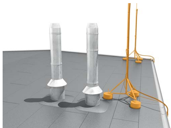
Рис. 2.70: Молниеприемные мачты isFang с расположенным снаружи токоотводом isCon®
