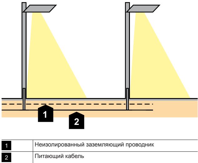
Рис. 3.26 Проводка кабеля
