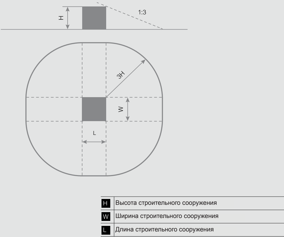
Рис. 1.22: Эквивалентная область захвата прямых ударов молнии
