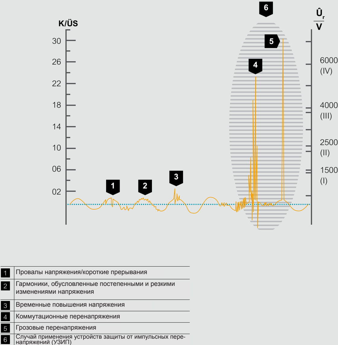
Рис. 1.8: Типы перенапряжений
