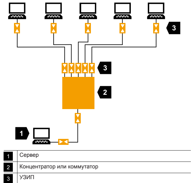
Рис. 3.34: Звездообразная топология
