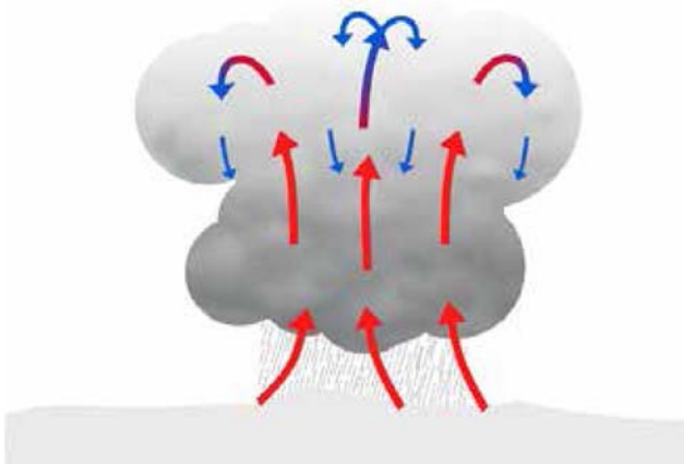
Рис. 1.4: Тепловая гроза
