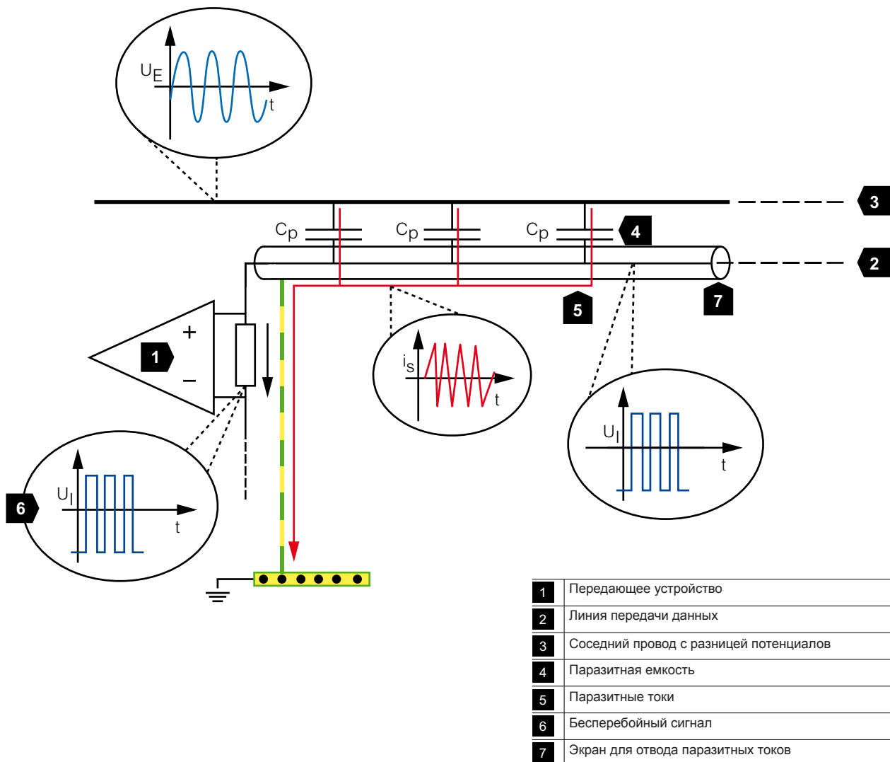
Рис. 3.47: Заземленный с двух сторон экран кабеля
