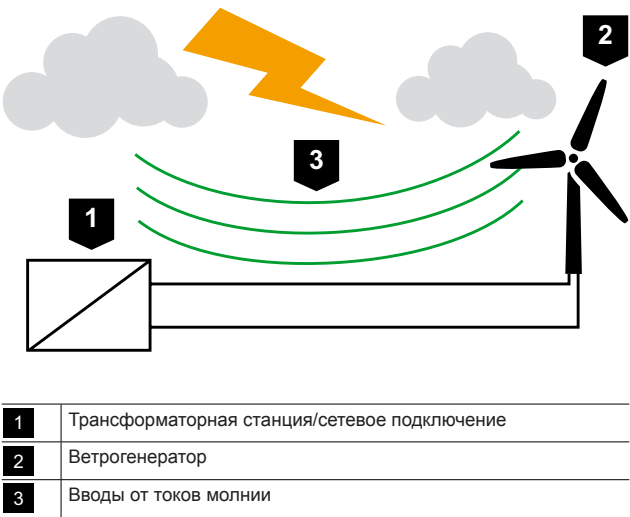
Рис. 3.21: Меры молниезащиты и защиты от импульсных перенапряжений ветрогенераторов
