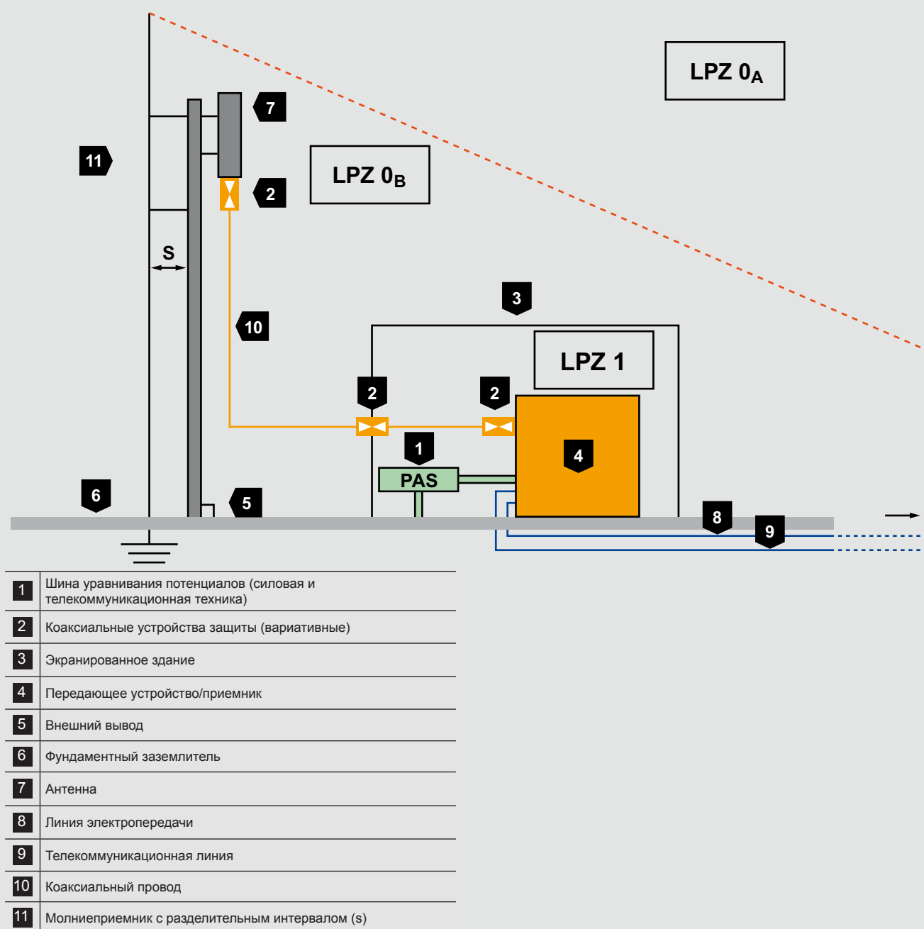
Рис. 3.77 Защита антенной установки
