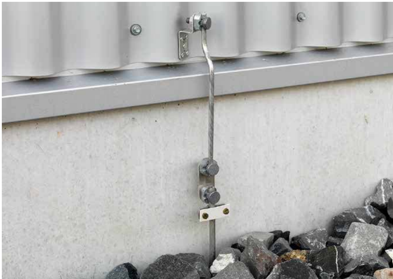
Рис. 4.1: Место разделения на металлическом фасаде
