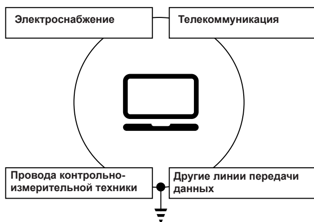
Рис. 3.20: Цепь защиты вокруг электрического прибора
