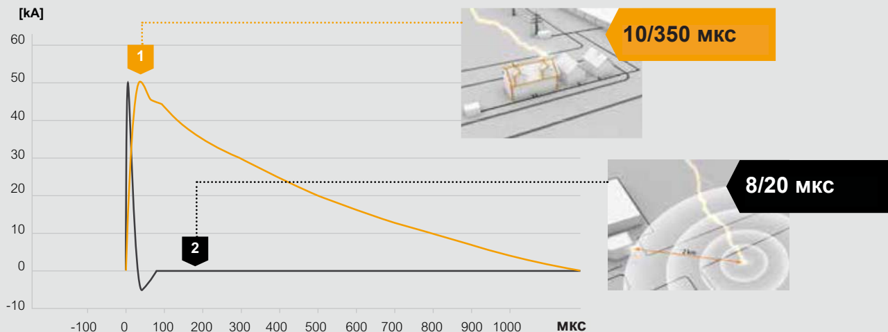
Рис. 1.15: Виды импульсов и их характеристика
