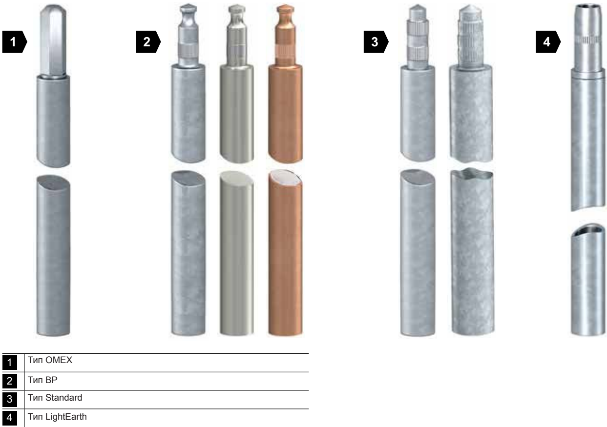
Рис. 2.87: Варианты глубинных заземлителей
