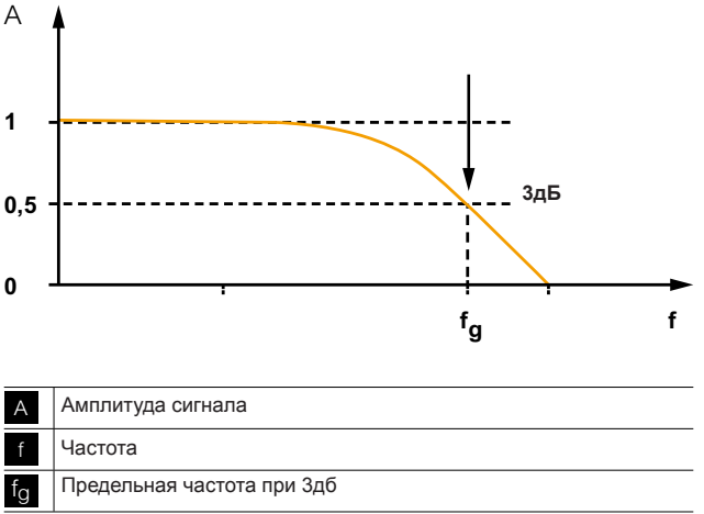
Рис. 3.53: Предельная частота f_n
