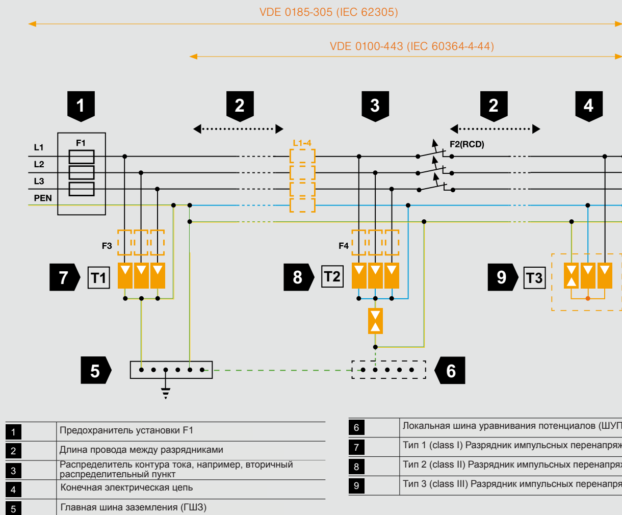
Рис. 3.11: 4-проводниковые сети, сетевая система TN-C и область применения стандартов
