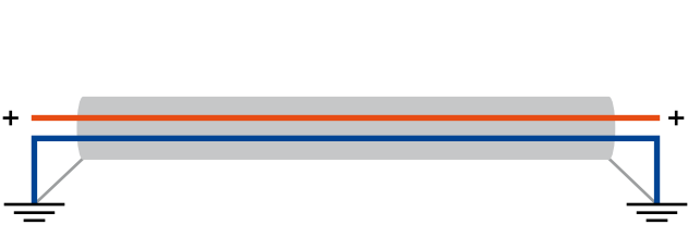
Рис. 3.53 Асимметричный провод
